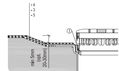
3.2. b bitumenes lemezből készült fólia csatlakoztatásának részlete
