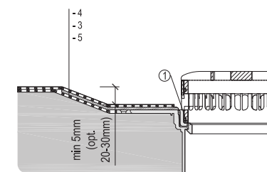
3.2.b Detaliu conexiune folie din benzi de asfalt
