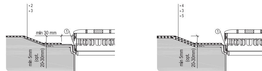
3.2.a Detail napojení fólie mPVC (TPO-FPO)
