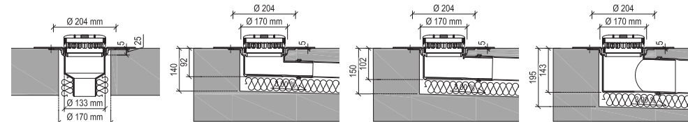
Воронка для террас вертикальная DN 70, 100, 125
