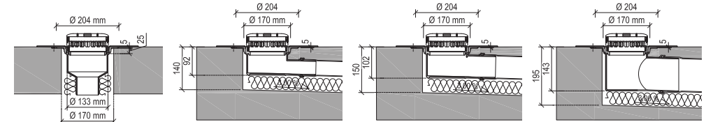
függőleges teraszösszefolyó DN 70, 100, 125
